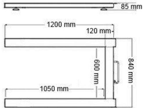
Croquis de las dimensiones de la balanza para pales
